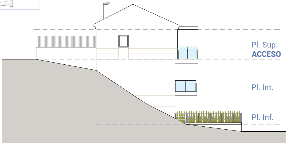
Alzado sur South elevation
