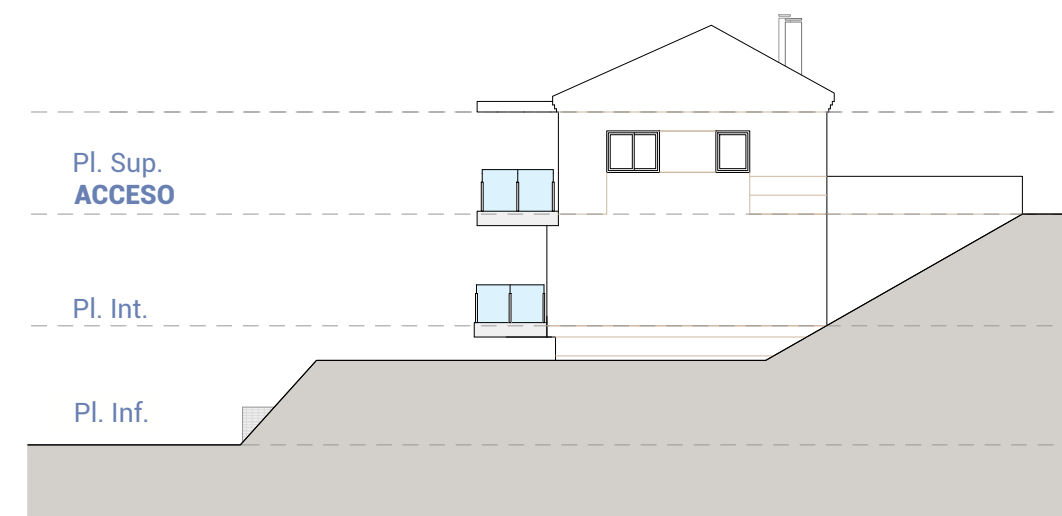
Alzado este East elevation
