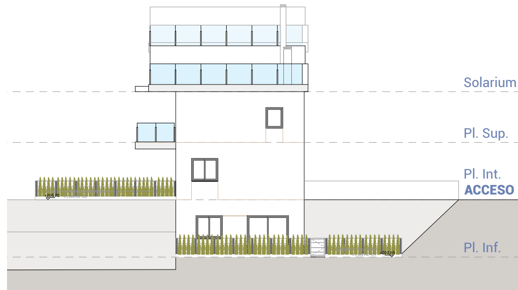
Alzado este East elevation
