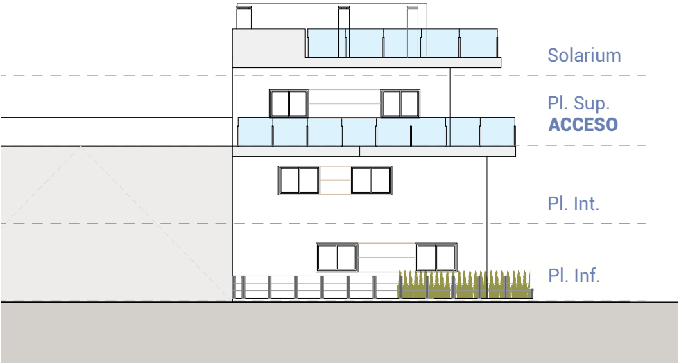
Alzado sur South elevation
