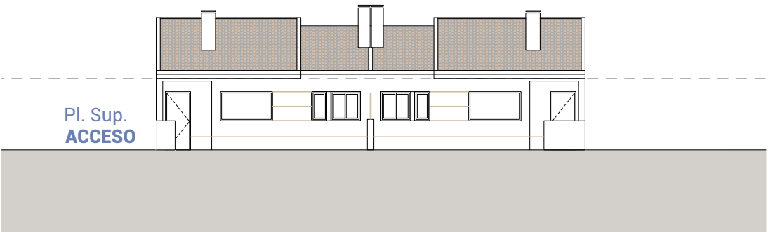
Alzado oeste (Calle Serra Gelada) West elevation (C/ Serra Gelada)
