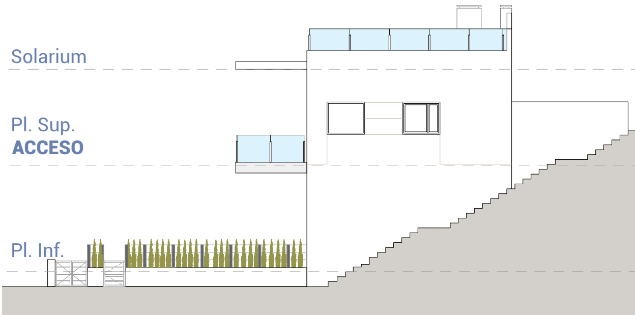
Alzado este East elevation
