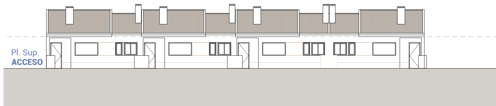
Alzado norte (Calle Serra Gelada) North elevation (C/ Serra Gelada)
