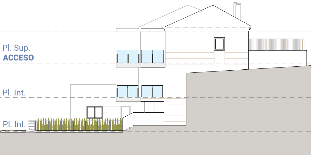
Alzado este East elevation
