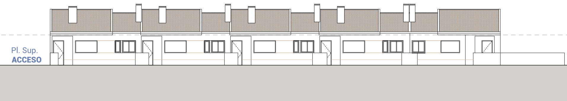
Alzado norte (Calle Serra Gelada) North elevation (C/ Serra Gelada)
