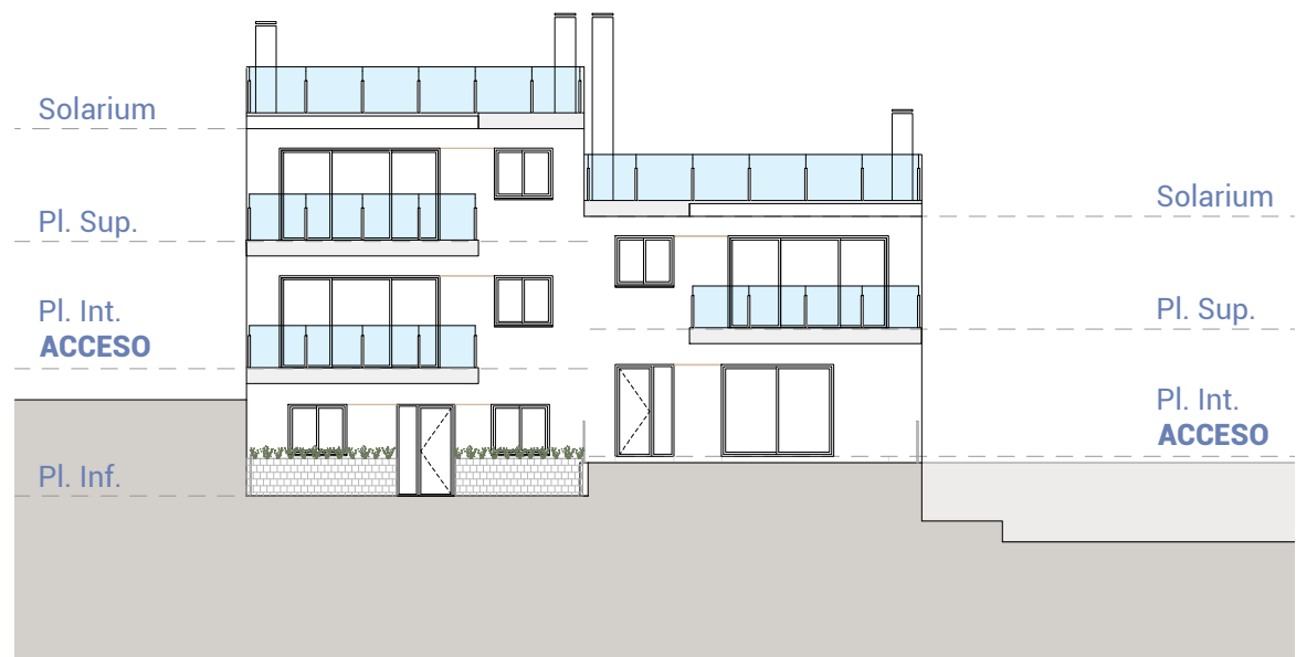
Alzado sur (Jardines privados) South elevation (Private gardens)
