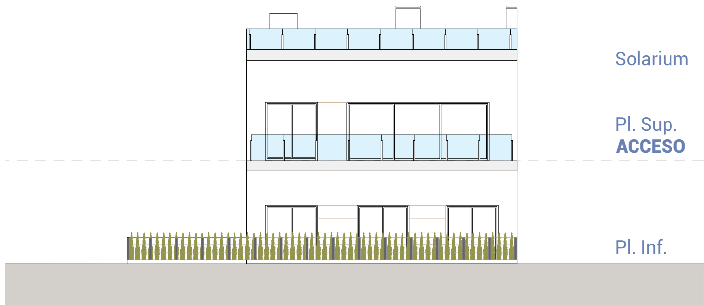
Alzado sur (Jardines privados) South elevation (Private gardens)
